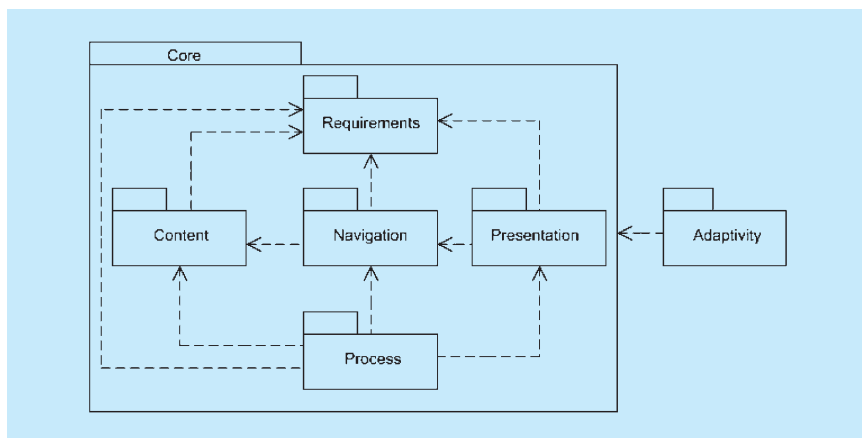
Bild 8: UWE-Metamodell
